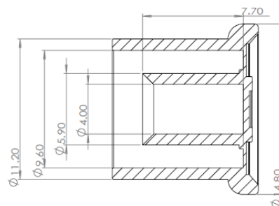
剖面 A-A
